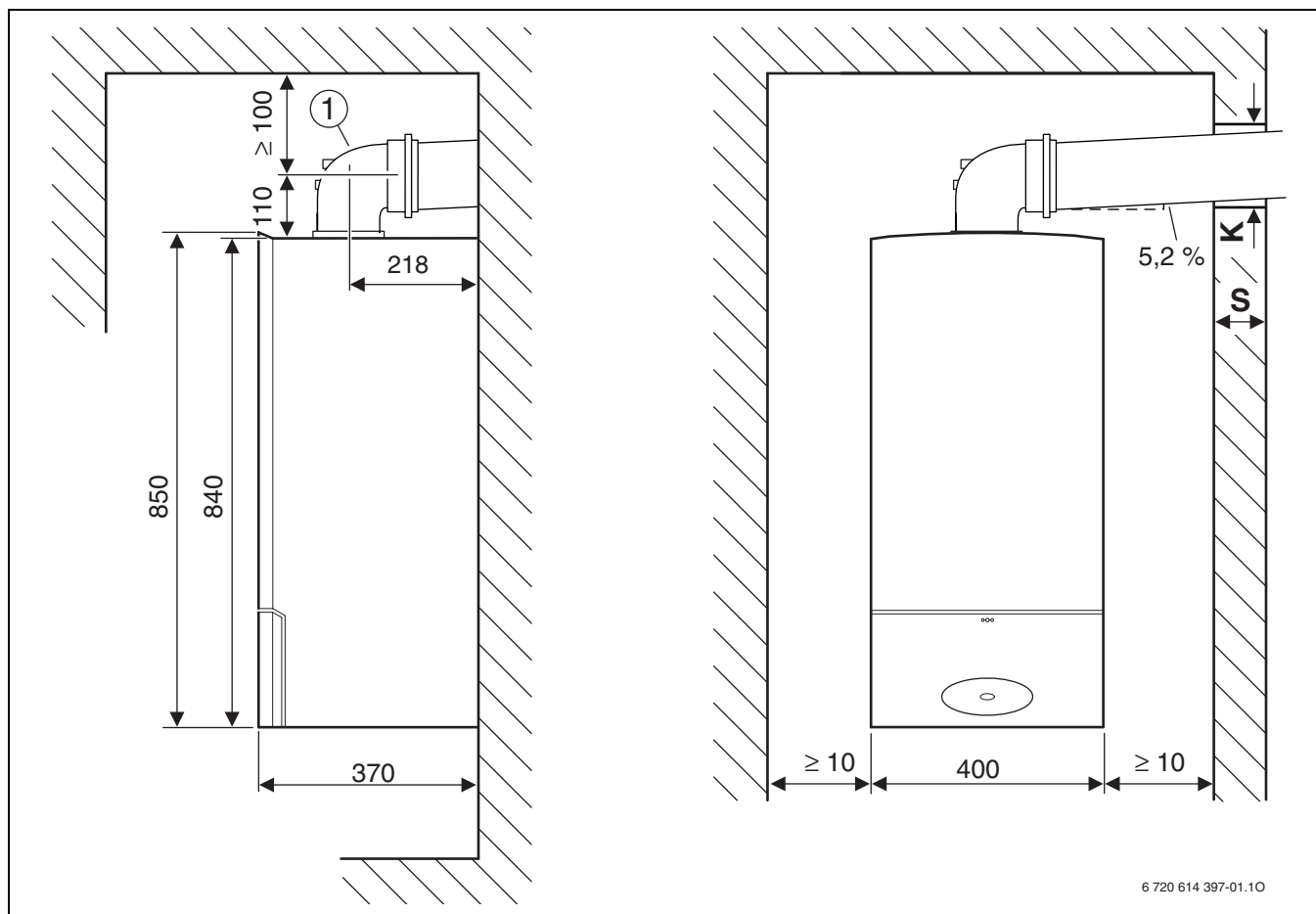
Joon. 5 Suitsugaasi juhtimine Ø 80/125 mm või Ø 80 mm
