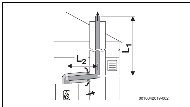
Joon. 31 Jäik heitgaasi juhtimine šahtis tarvikusse B 53p ruumi õhust sõltuva õhu juurdevooluga kontsentrilise õhu ja heitgaasi juhtimise kaudu katlaruumis
