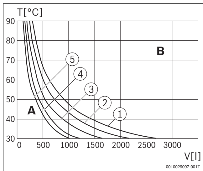
Joon. 42 Paisupaagi karakteristikud (29 I)
